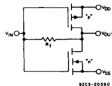
Fig. 5—COS/MOS amplifier.
