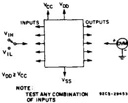
Fig. 14 - Input voltage.
