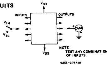
Fig. 10 - Input voltage.
