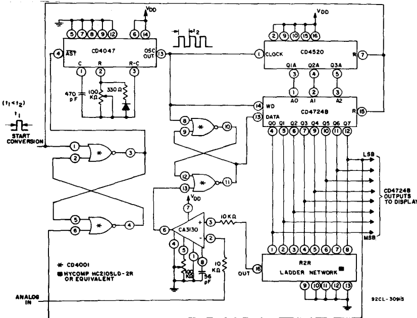
Fig. 5—A/D converter
