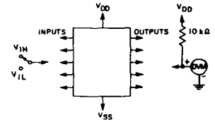
Fig. 10 - Input-voltage test circuit.
