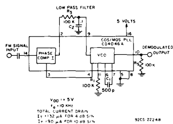
Fig. 10— FM demodulator.
